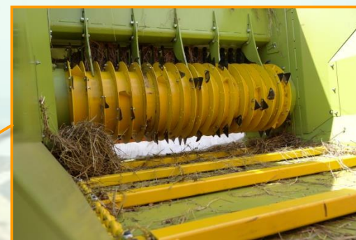
Ревёрсивный цепной транспортер
