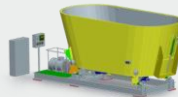
Стационарные смесители кормов. ССК от 12м 3 до 30м 3
